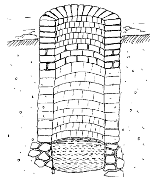
Puits entièrement revêtu
